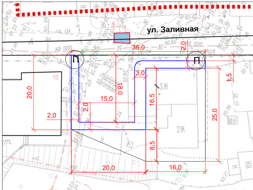
Понижение бордюрного камня (П)
